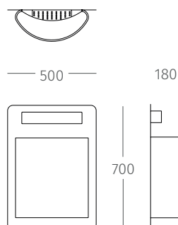
Metro Abfallbehälter mit Aschenbecher
