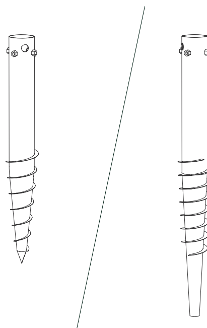
Schraubfundament 800 oder 1000 für 5 kN: 800; für 15 und 30 kN: 1000
