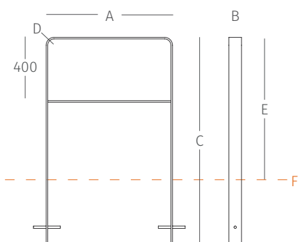
Clean R Fahrradständer zum Einbetonieren, mit Knieholm
