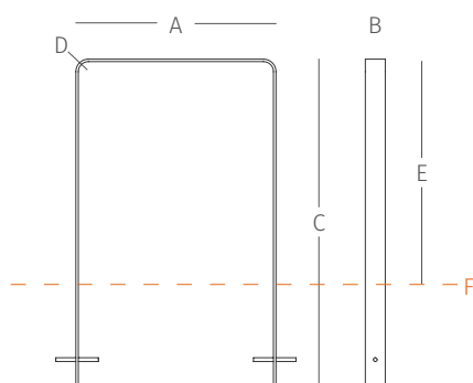
Clean R Fahrradständer zum Einbetonieren, ohne Knieholm
