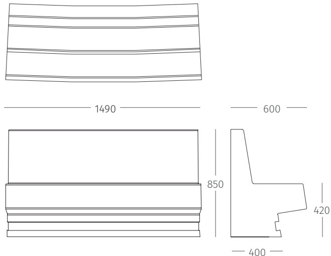
Bequer konvex, r = 14,7\text{ m}
