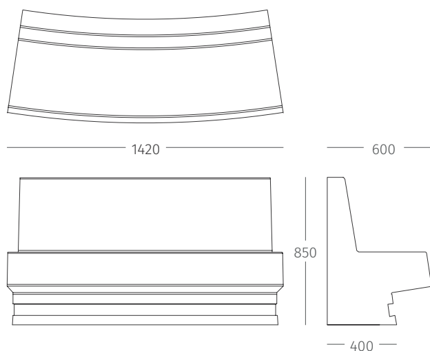
Bequer konvex, r = 4,7\text{ m}
